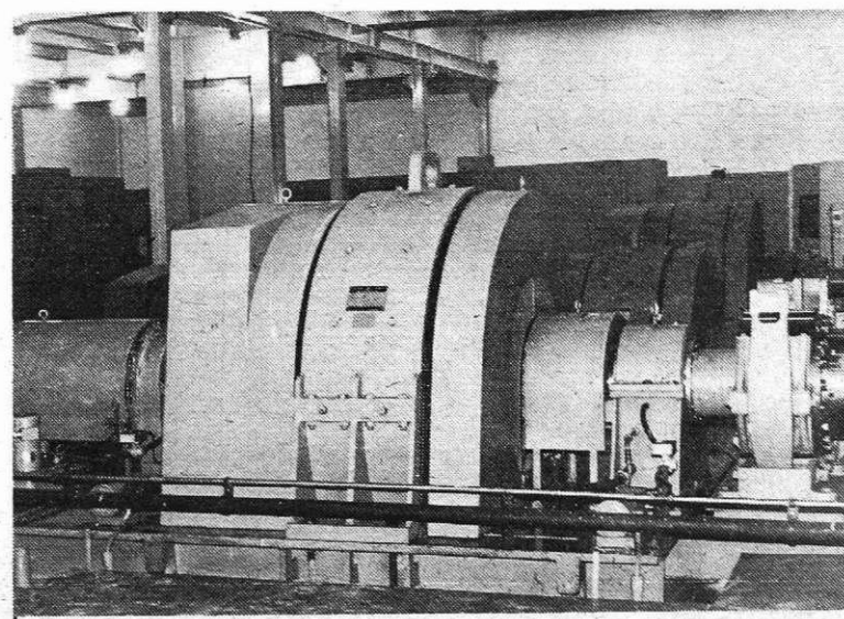
Strojnica Sendzimir ogrođa v hladni valjarni Bela
