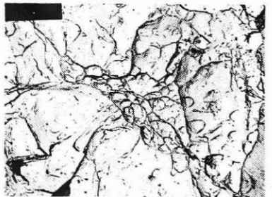
Frakto-grafska preiskava; kombinacija žilavega in krhkega loma pri 7.500 kratni povečavi (5)
