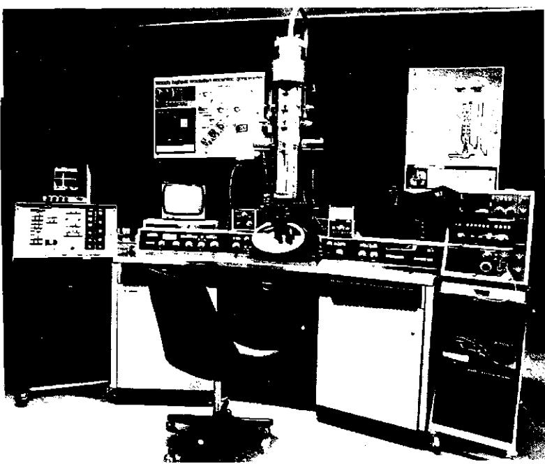
Elektronski mikroskop Philips z rentgenskim spektrometrom in scanning na pravo, instaliran v raziskovalnem oddelku (1)
