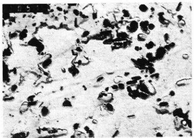
Izločki cementita v poboljšanem jeklu krat 36.000 (4)
