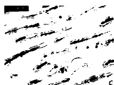
Primer modificiranega cementita pri 98.000 kratni povečavi (3)
