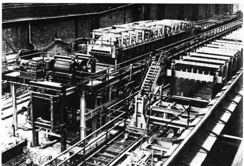
Lužilna linija za oglikova jekla z delom lužilne linije za nerjavna jekla v novi hladni valjarni
