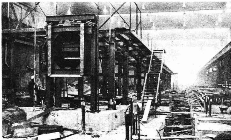
Podporna konstrukcija SCAP v novi hladni valjarni
