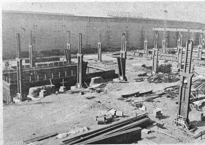
Temelji za novo žarilno peč v novi hladni valjarni
