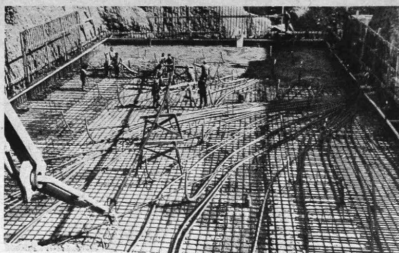
Betoniranje temeljev za zvonaste peči v novi hladni valjarni
