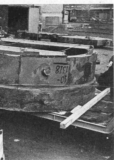
»Prsten« za cementarno Usje so odšli naši sodelavci v livarno. Premer »prstena« je okrog štiri metre, en kos pa tehta bruto 28 ton. Odlitek dokončno obdelajo v ljubljanskem Litostroju, kjer imajo za to ustrezne stroje.
