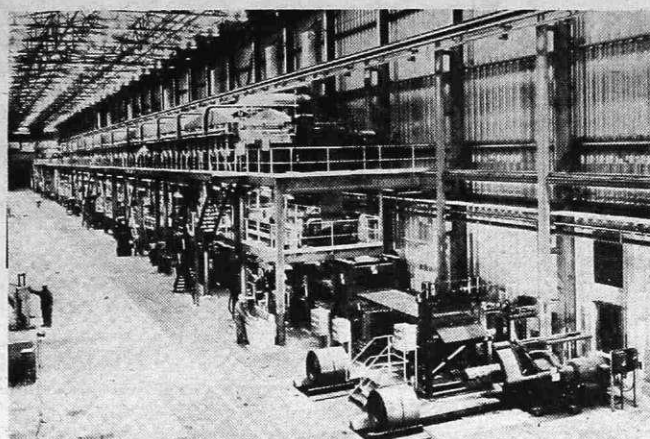
Žarilno-lužilna linija za dinamo trakove
