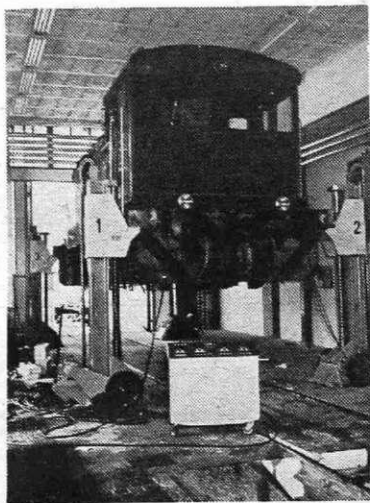
Nova lokomotivska delavnica v transportnih obratih, je opremljena z dvigalkami za dviganje lokomotiv, kadar je treba obnovljati njihovo podvozje. Zaradi popravil vozniških podstavkov, sedaj ni treba več lokomotiv pošiljati v Zagreb, kar je pomemben napredek pri hitrejšem in cenejšem vzdrževanju železniških vlečnih vozil.
