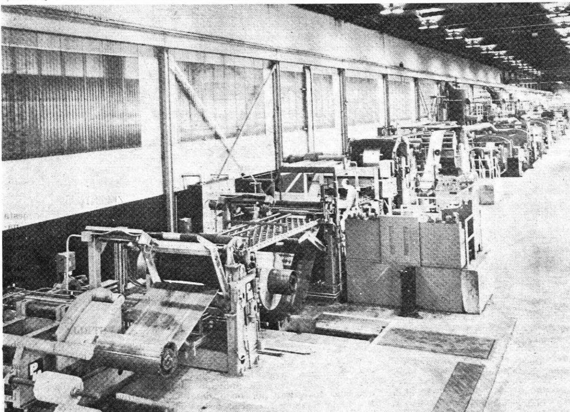
Razoglaševalno žarilna linija za dinamo trakove (foto arhiv »Production Machinery Corporation«)
