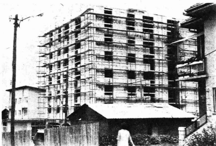
Stolpič za monterje nove hladne valjarne, ki ga gradijo delavci SGP Sava na Koroški Beli, je pod streho. V njem bo 53 garsonjer, v pritličju kuhinja, restavracija, bife, mesnica in samopostrežna trgovina TP Žarja TOZD Delikatesa. Po dograditvi hladne valjarne bodo garsonjere z manjšimi adaptacijami preuredili v družinska stanovanja. Predvidevajo, da bosta do zaključka septembra prvi dve etaži garsonjer gotovi, druge pa bodo izgovarjali postopoma.
