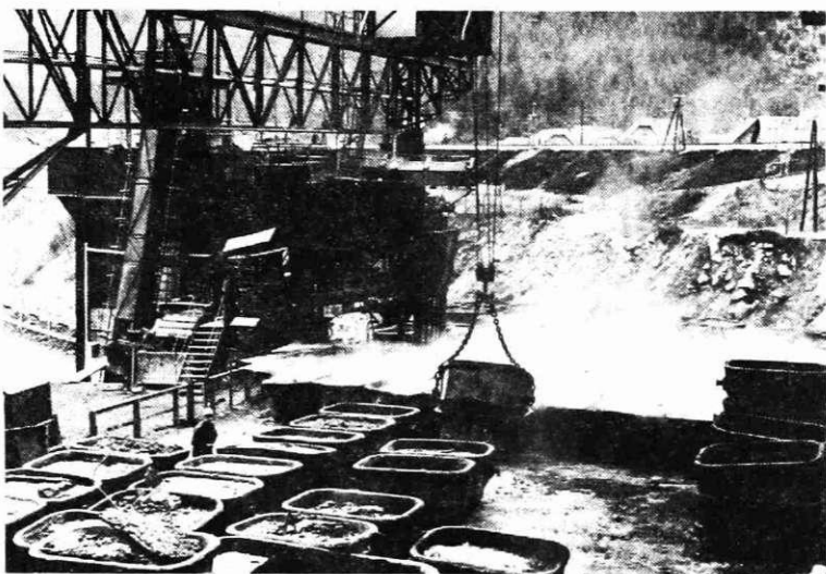
Predelava žlindre v kosovno
