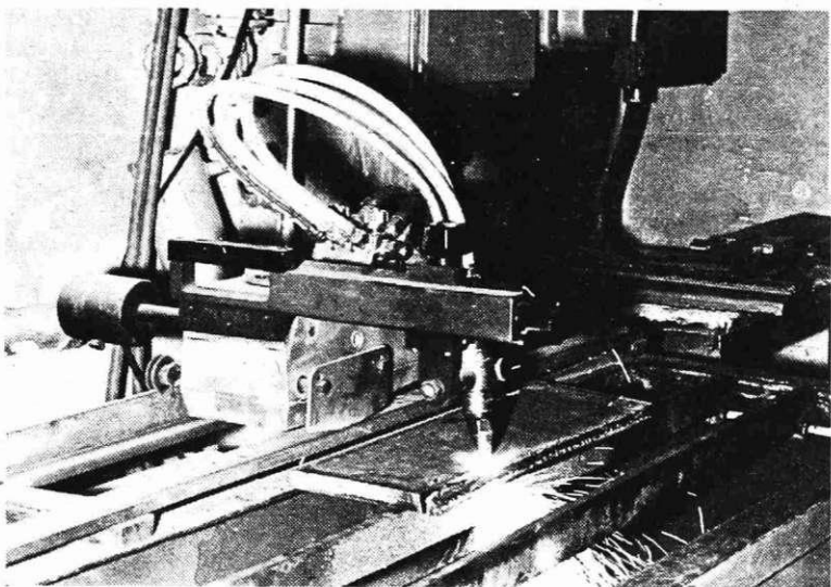
Slika 3: Sekator med delom
