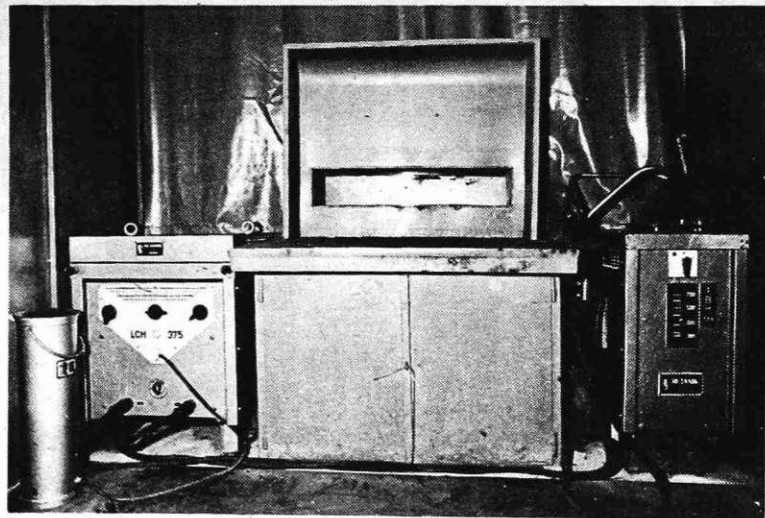
Slika 1: Varilna kabina z usmernikom in transformatorjem
