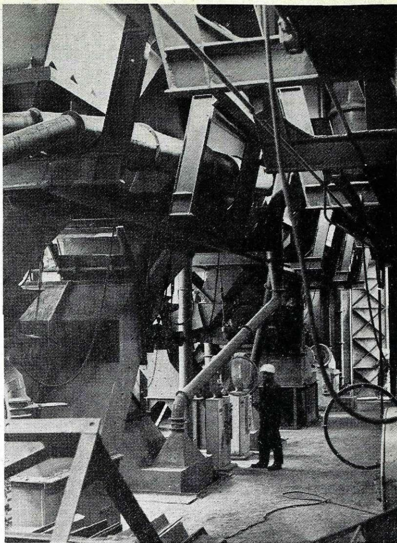
Aglomeracija, objekt 30 — silosi za sinterizirano rudo
