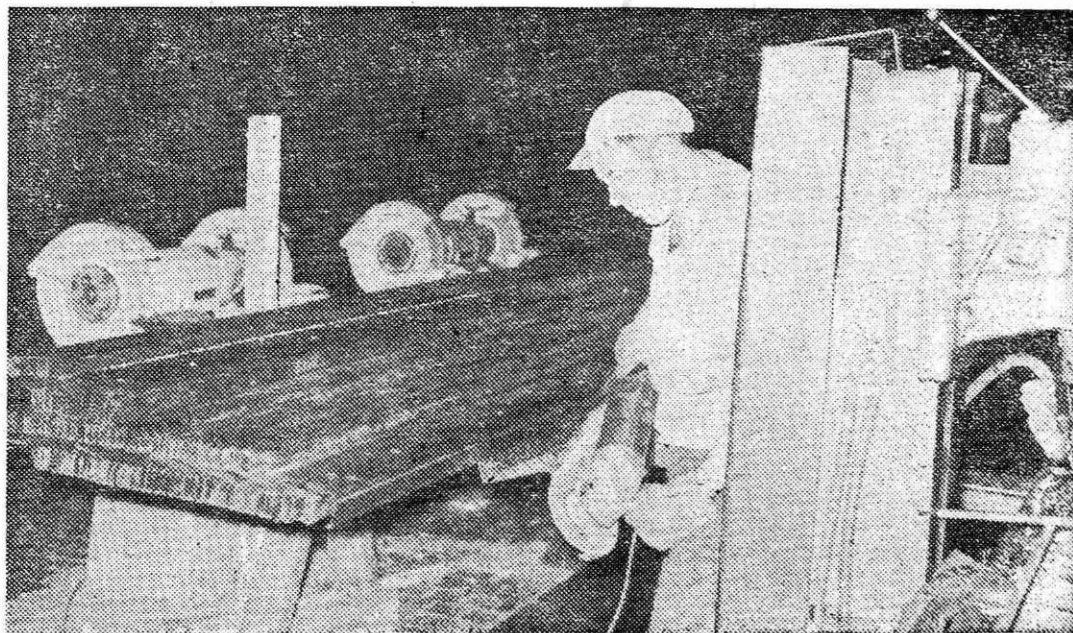
Brušenje profilov v profilarni
