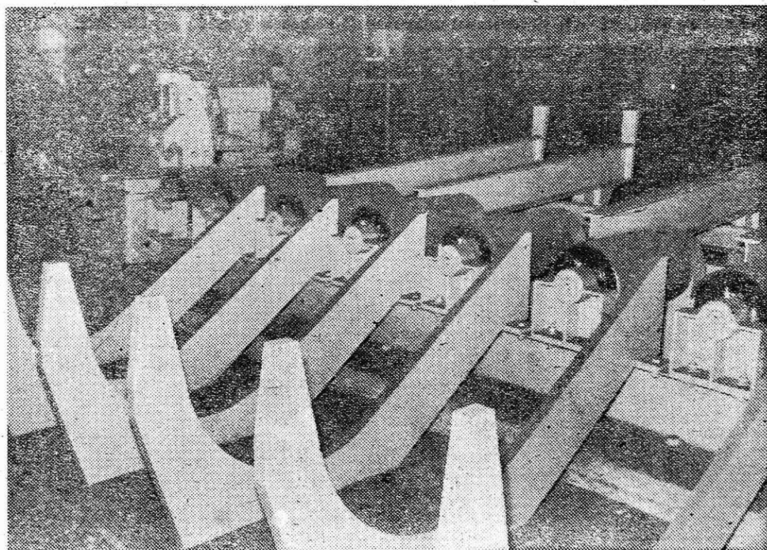
Stroj za rezanje vzorcev (prob) v tretji hali valjarne Bela
