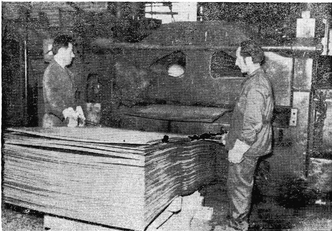
Ravnalni stroj v adjustaži štekel na Javorniku
