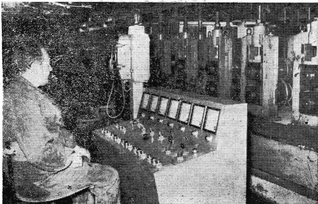
Sodelavec pri komandnem pultu na oblikovalni progi ROSSI v profilarni
