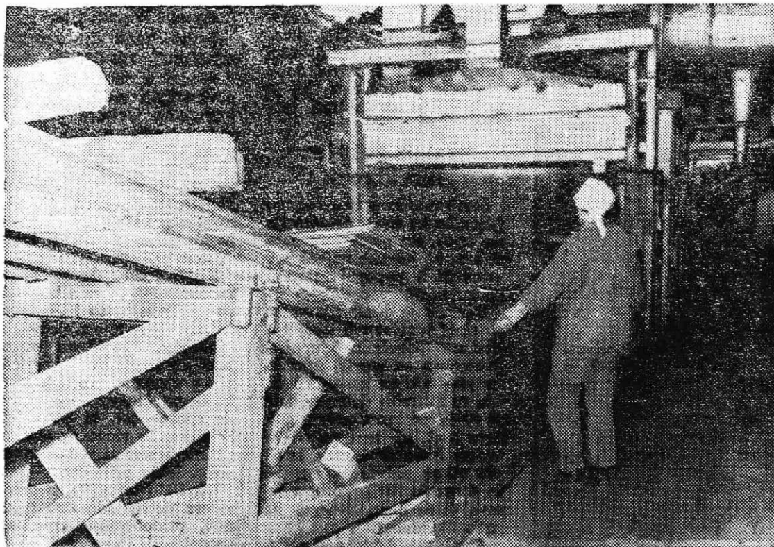
Normalizirna peč na Javorniku — ogrevana s propan-butanom
