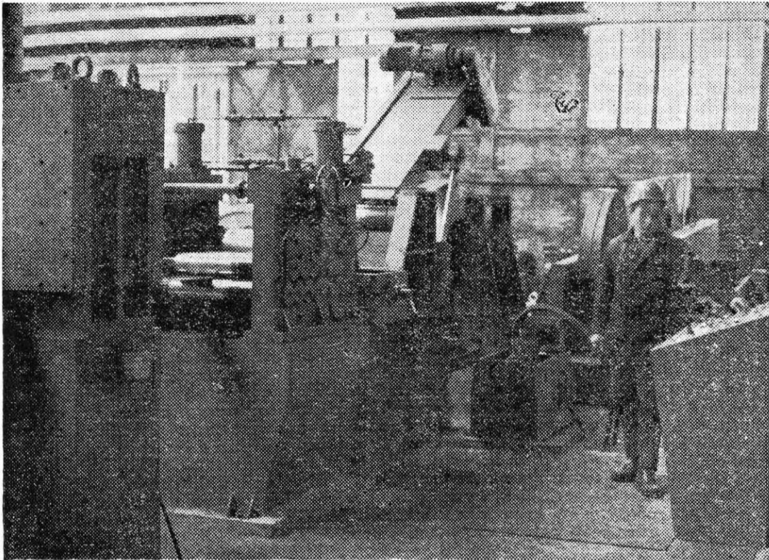
Del oblikovalnega stroja v novi profilarni na Javorniku
