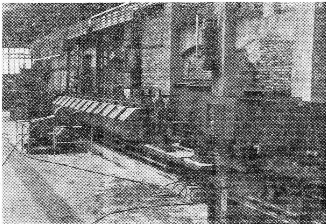
Del naprav za proizvodnjo hladno valjanih profilov v novem obratu na Javorniku
