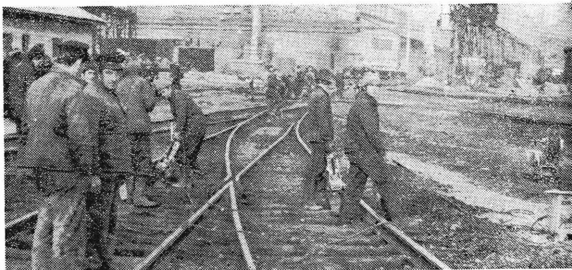
Namesto lopat in krampov, smo dobili mehanizirane podbijalke za podbijanje pragov
