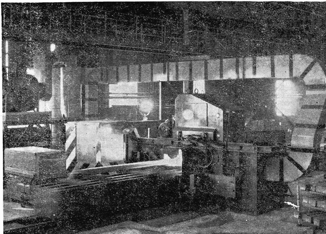
Valjarna Bela, naprava za plamensko čiščenje bram
