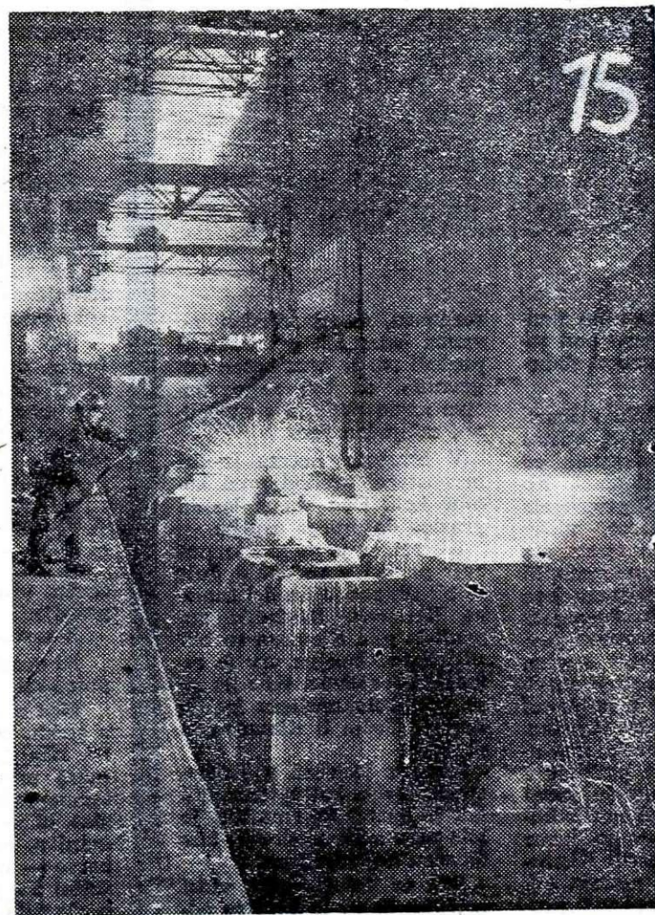
Žerjavi v livni jami martinarne
