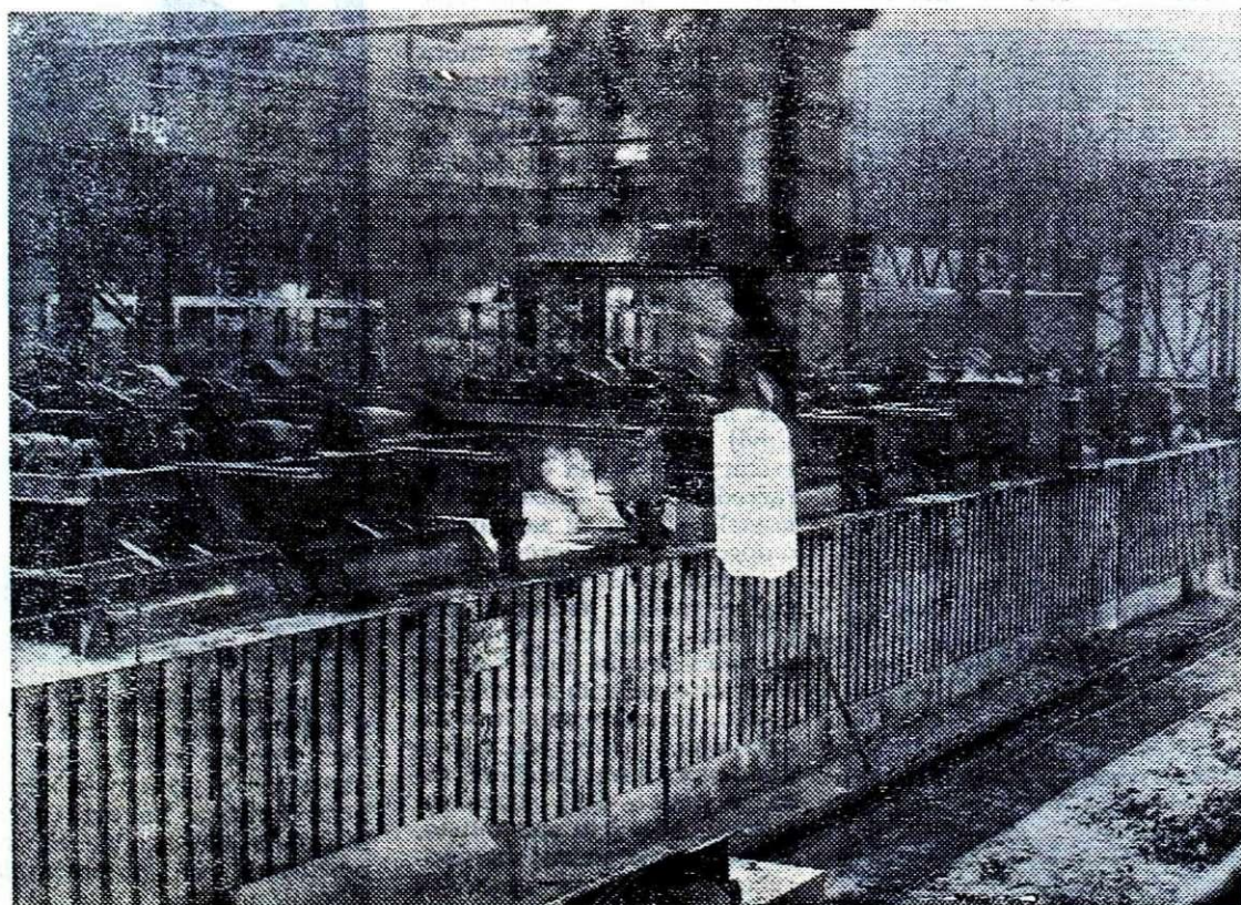
Kleščni žerjav dviga iz globinske peči ingote ali brame
