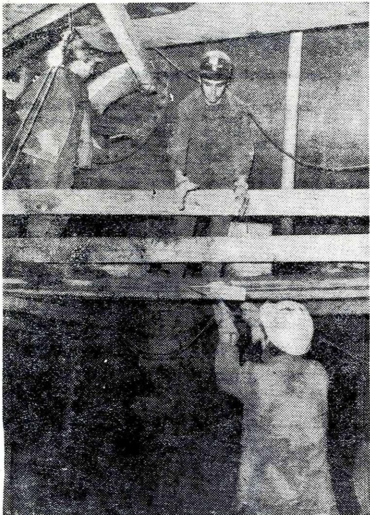
Zidarji Vatrostalne zaključujejo obzidavo nove venčne cevi z zapiranjem vstopne odprtine
