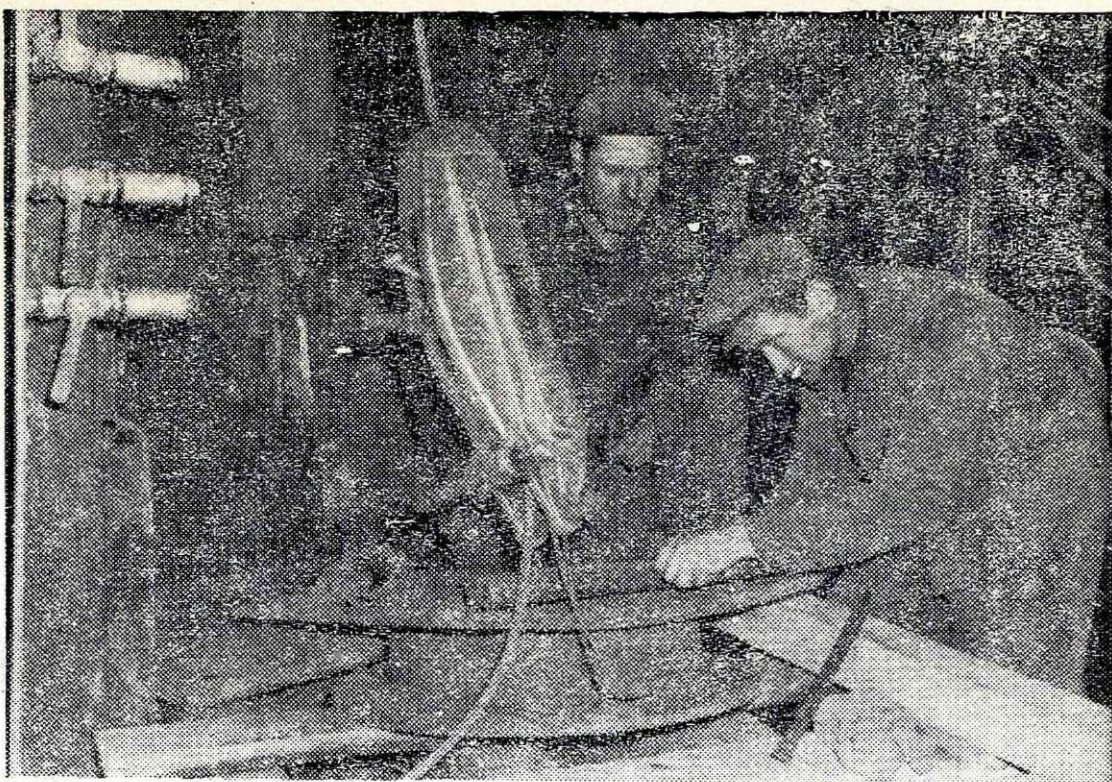
Monterja Metalne bosta zaprla zadnjo odprtino na plašču talilnika z namestitvijo žlindernice
