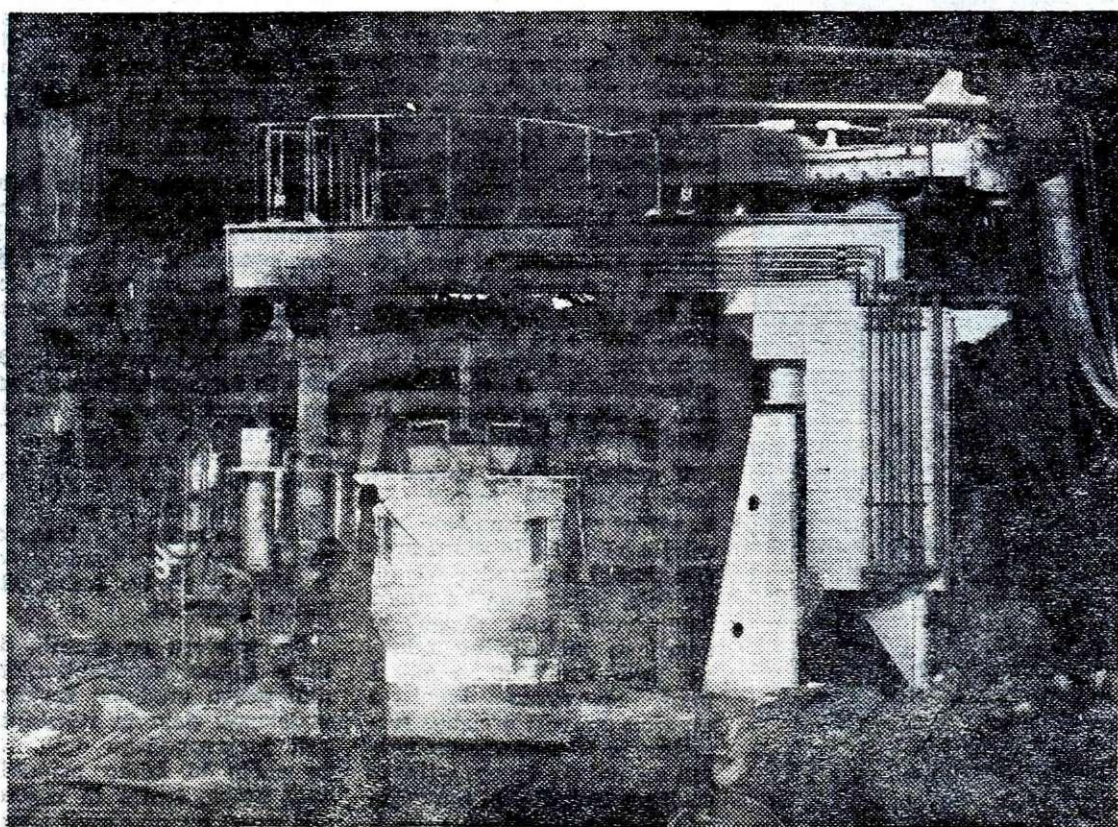
Električna peč po letošnjem generalnem remontu
