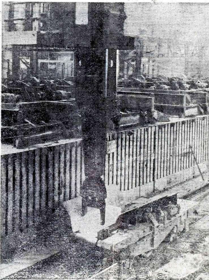
Ingot na transportnem vozičku pripravljen za valjanje
