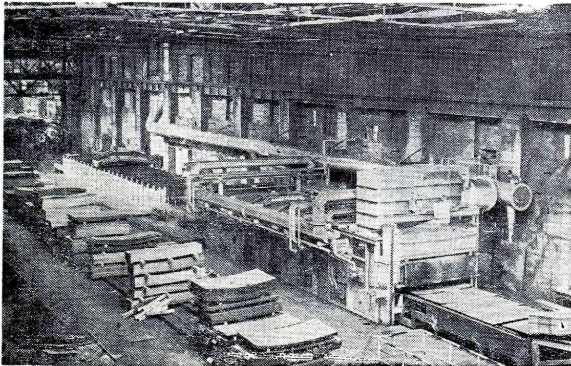
Normalizirna peč v valjarni na Javorniku
