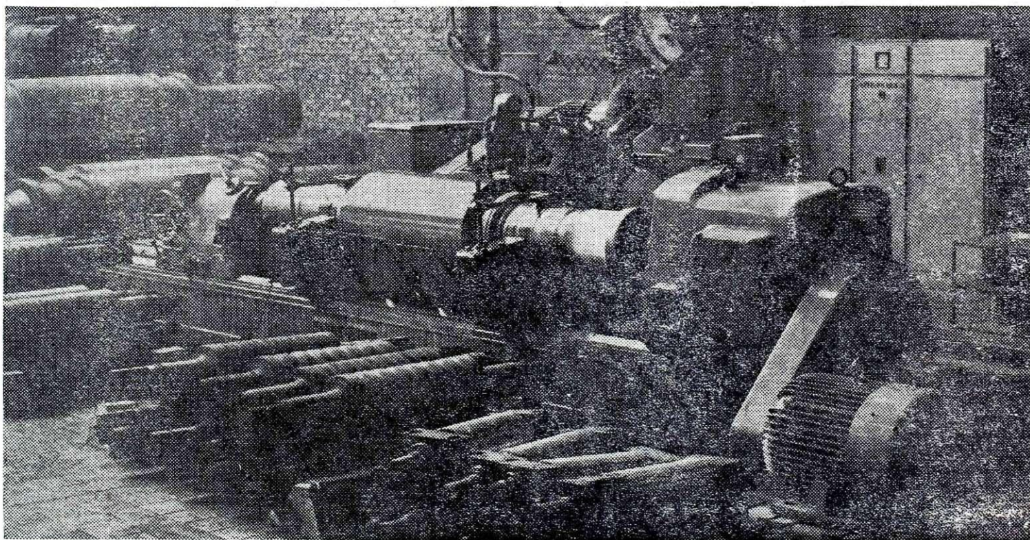
Sodelavec pri stružnici valjev v valjarni Bela
