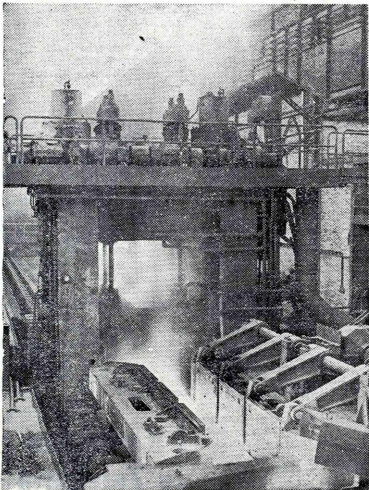
Bluming valjarna na Beli
