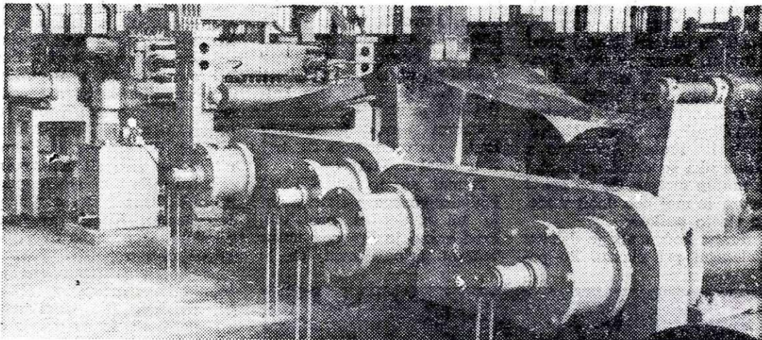
Konti peč v rednem obratovanju
