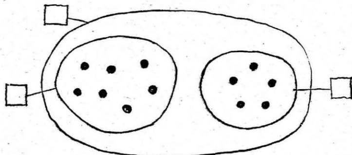
ZDRUŽENA MNOŽICA (unija)
