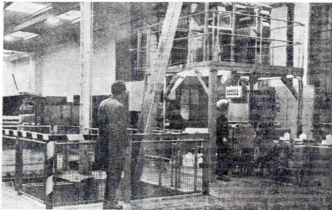
WAFIOS pakirni stroj v žebljarni
