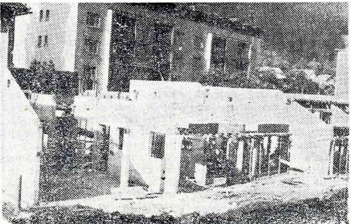
Gradnja nove zgradbe za vrtec na Plavžu dobro napreduje. Kot vidimo na sliki, bo paviljonska zgradba sestavljena iz posebnih elementov. Dela opravljajo delavci SGP Sava. — V novi stavbi bo skupaj s prenovljeno staro stavbo, prostora za 160 varovancev, od katerih bo lahko tudi 20 dojenčkov. Računajo, da bo vrtec zgrajen še letos. B.
