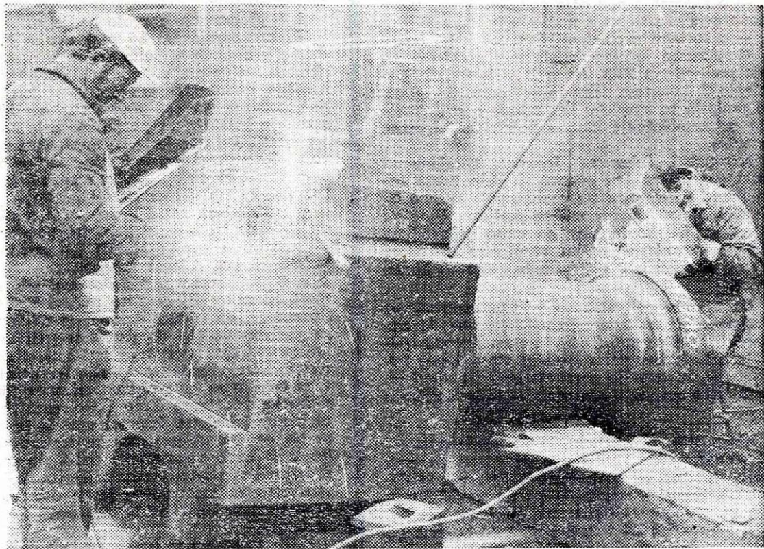
Obdelava večjega odlitka v livarni
