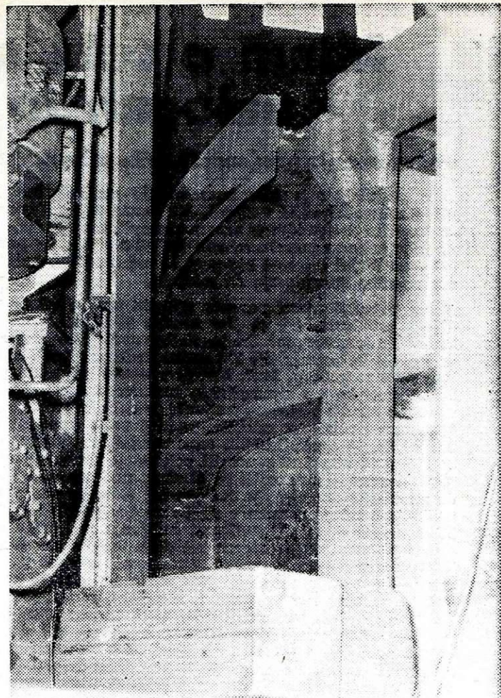
Lectromelt el. peč po eksploziji — pogled na pretrgani venec in izboklo steno
