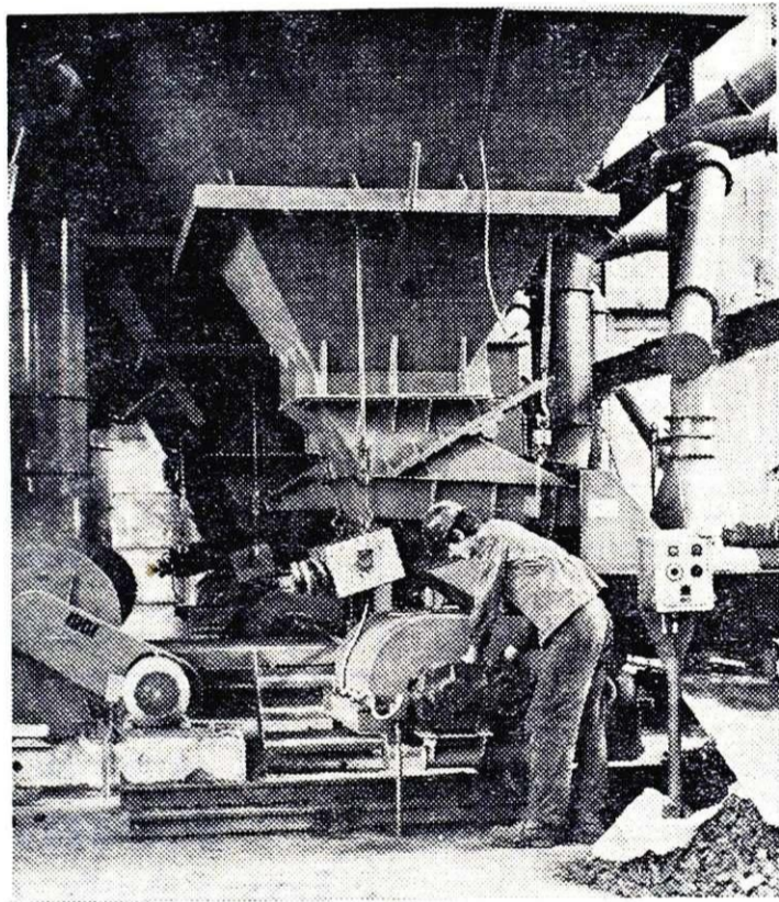
Silosilni apnenca in kokska z vibracijskimi dodajalci — aglomeracija
