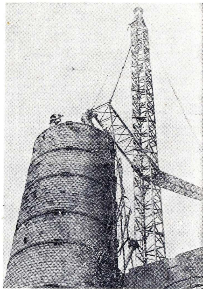
Rušenje dimnika starih ogrevalcev zraka na plavžu
