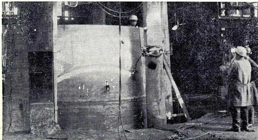
Montaža novega plašča talilnika na plavžu
