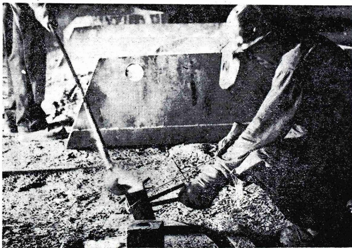
Vlivanje poskusnega jekla v martinarni
