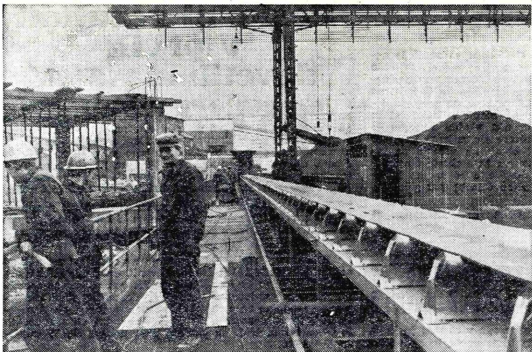
Izsek iz montaže naprav za novo aglomeracijo
