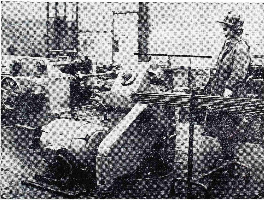
Ravnanje profilov na BLAW KNOX MEDART stroju v brusilnici na Javorniku
