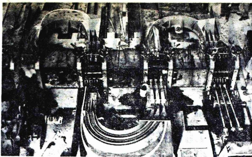
Proga 270 Ø s krožnimi vodili v novi valjarni žice na Belfi.
