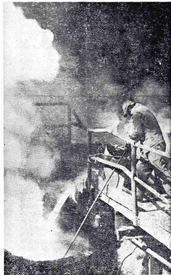
Remont plavža II. je bil od vseh remontov doslej izveden v najkrajšem času
