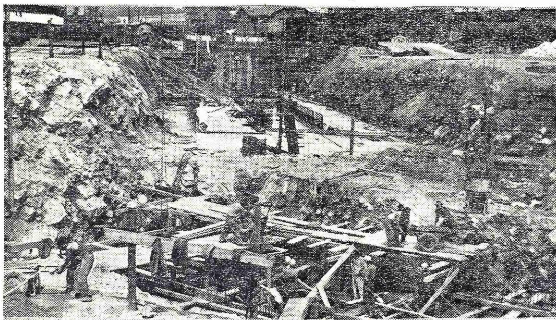
Danes obširneje poročamo o gradnji nove aglomeracije, katere del vidite tudi na tej sliki in sicer temelje za stolp v skladišču koksa, v ozadju pa stometrski rov
