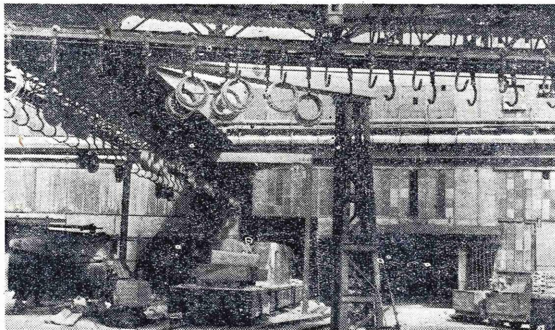
Brane in kokile z branami čakajo, da jih bodo prepeljali v valjarno Bela
