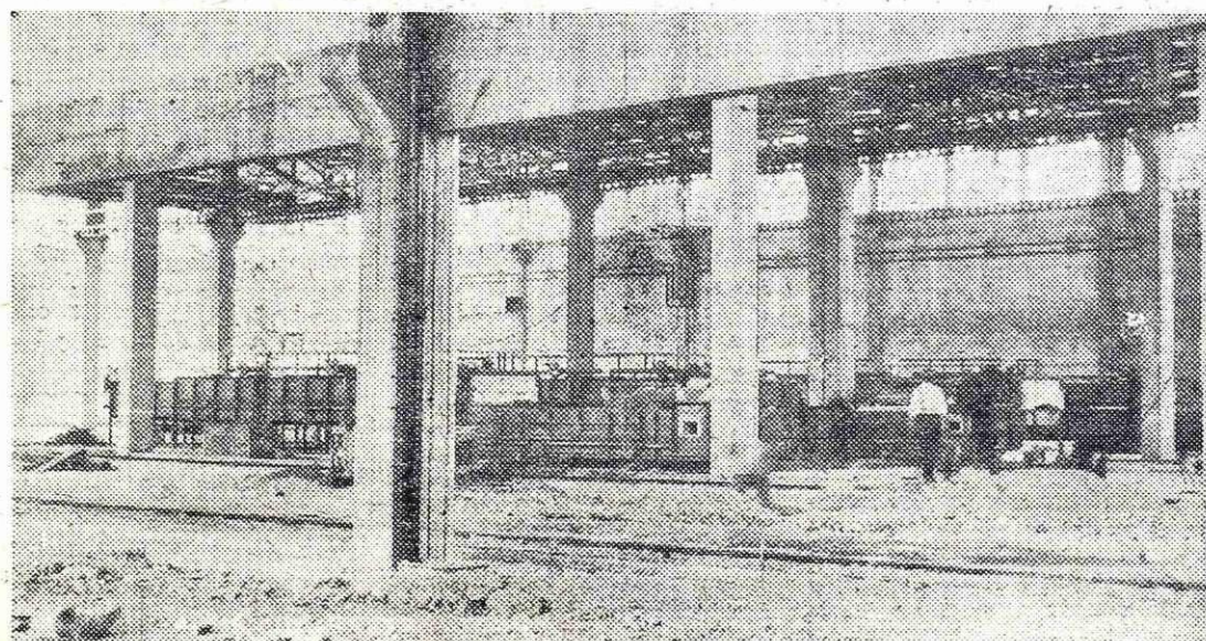
Poleg žičarne je zrasla nova hala — patentirnica. Dela so napredovala sedaj tudi v notranjosti in je oprema že pripravljena za namestitve
