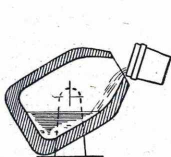
Posamezne faze procesa in obračanje konvertorja pri tem
