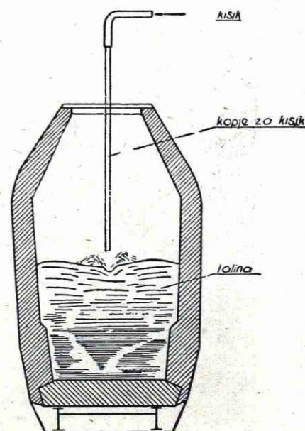
Skica LD konvertorja
