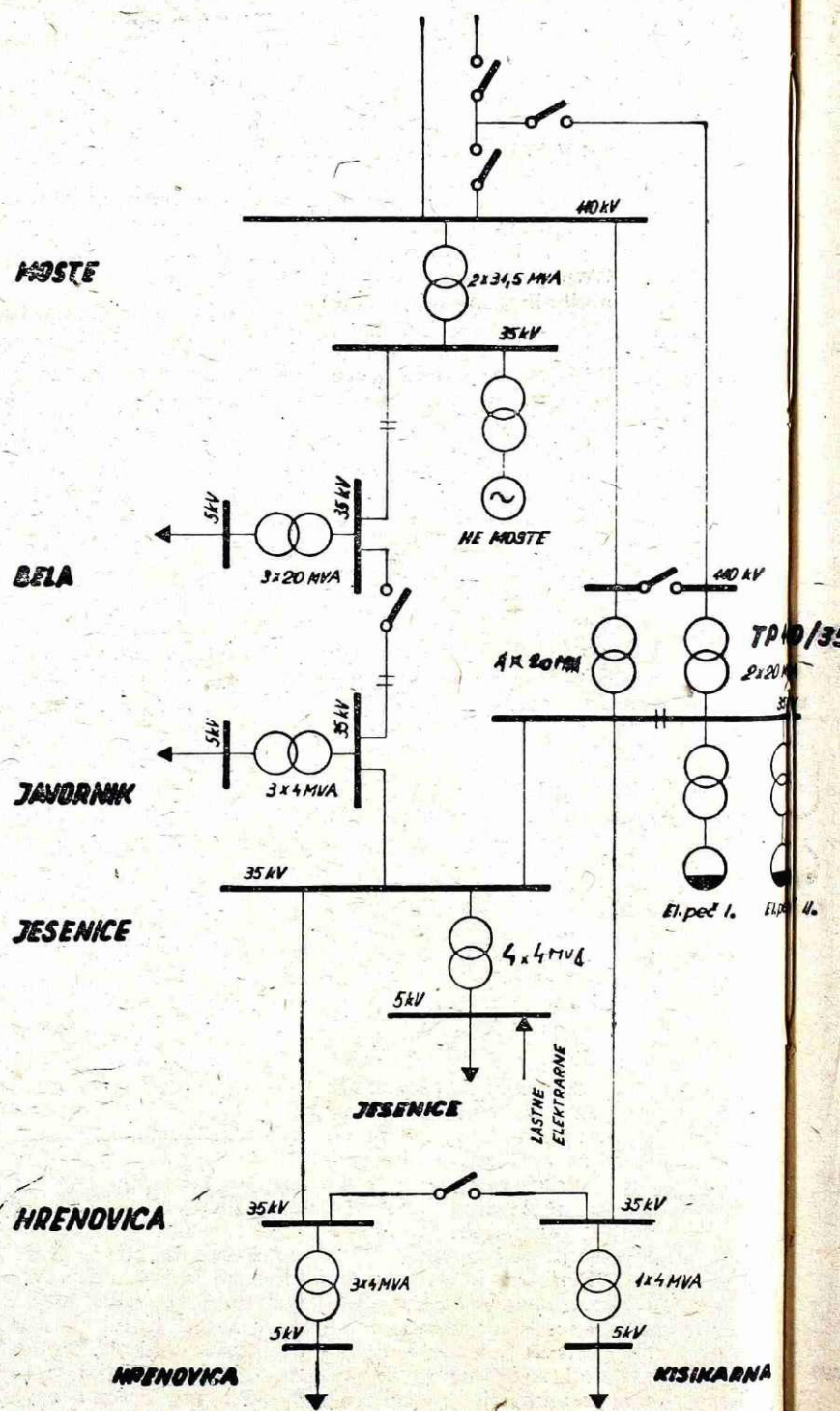
BODOČE NAPAJANJE NAŠE ŽELEZARNE
