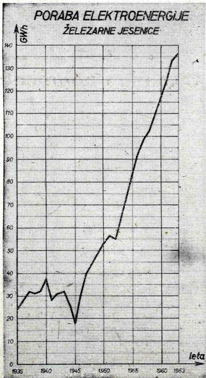
Naša železarna dobiva električno energijo iz HE Moste in Kleče. Na novi 110 kV d. l. rovod Jesenice—Moste, ki je že zgrajen, bodo priključene nove električne peči naše železarne. S tem je rešen problem nihanja napetosti na omrežju ELES.
