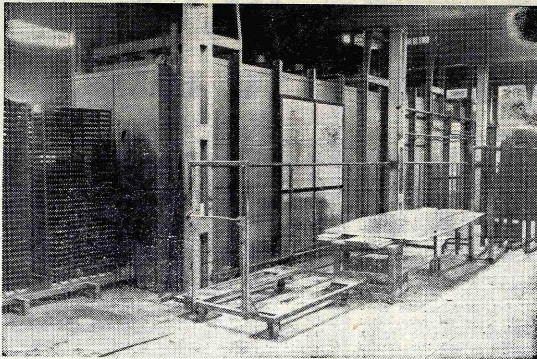
Z rednim obratovanjem nove sušilne peči bo v elektrodnem oddelku odpravljeno ozko grlo pri sušenju elektrod
