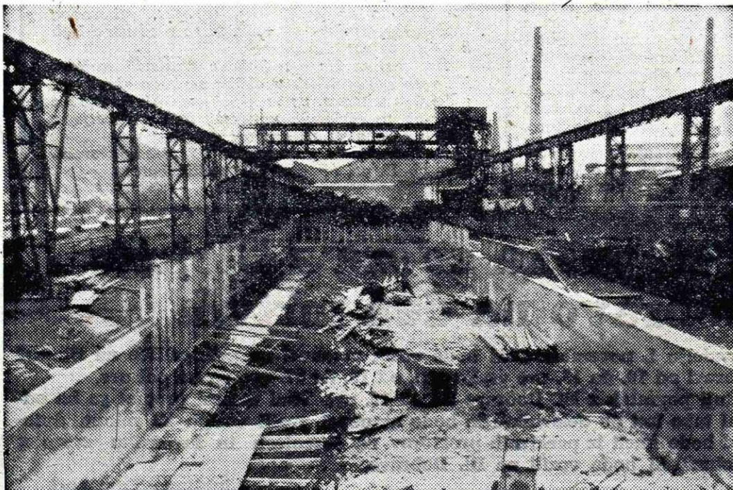
Na haldi pod Sava žerjavom so zgradili jamo za staro železo za novo električno peč.
