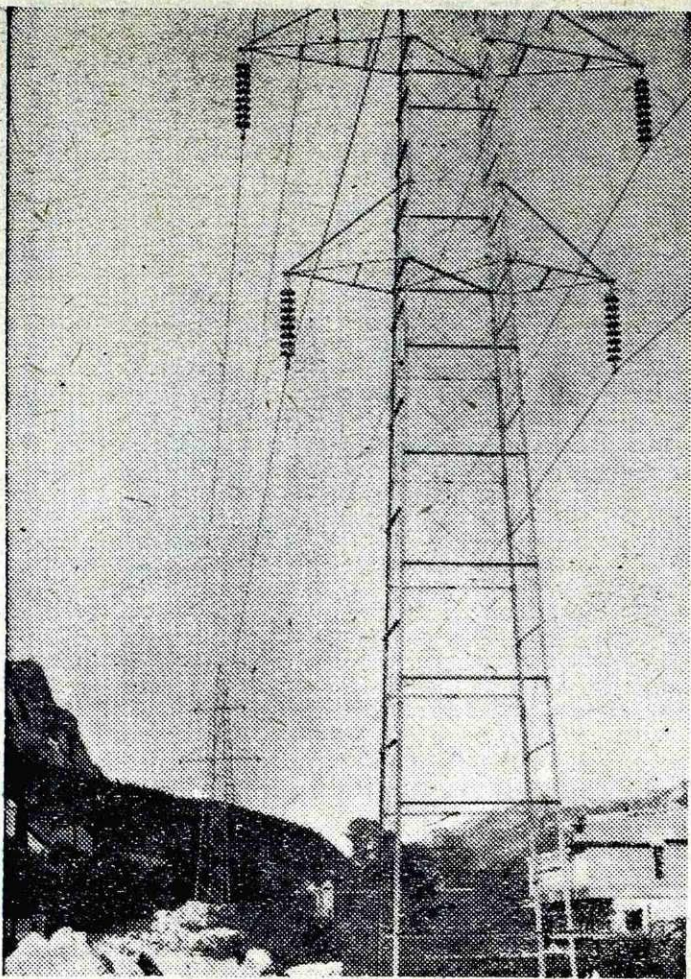
Naša železarna dobiva električno energijo iz HE Moste in Kleče. Na novi 110 kV d. l. rovod Jesenice—Moste, ki je že zgrajen, bodo priključene nove električne peči naše železarne. S tem je rešen problem nihanja napetosti na omrežju ELES.
