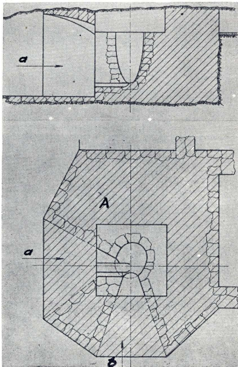
Plavž pri Koritih v preseku in tlorisu Foto S. Smolej
