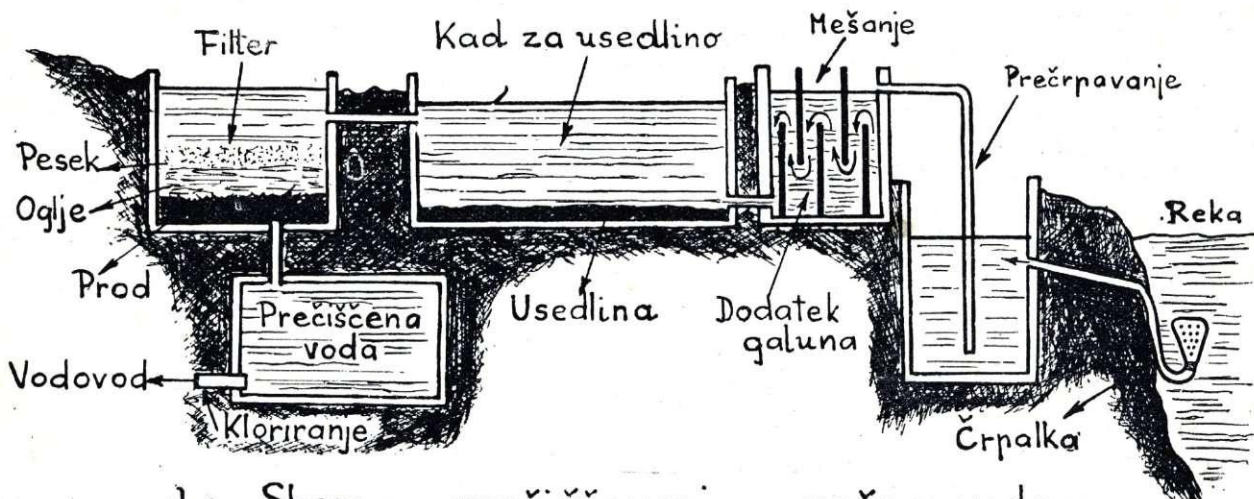
sl. 2. Shema prečiščevanja rečne vode
