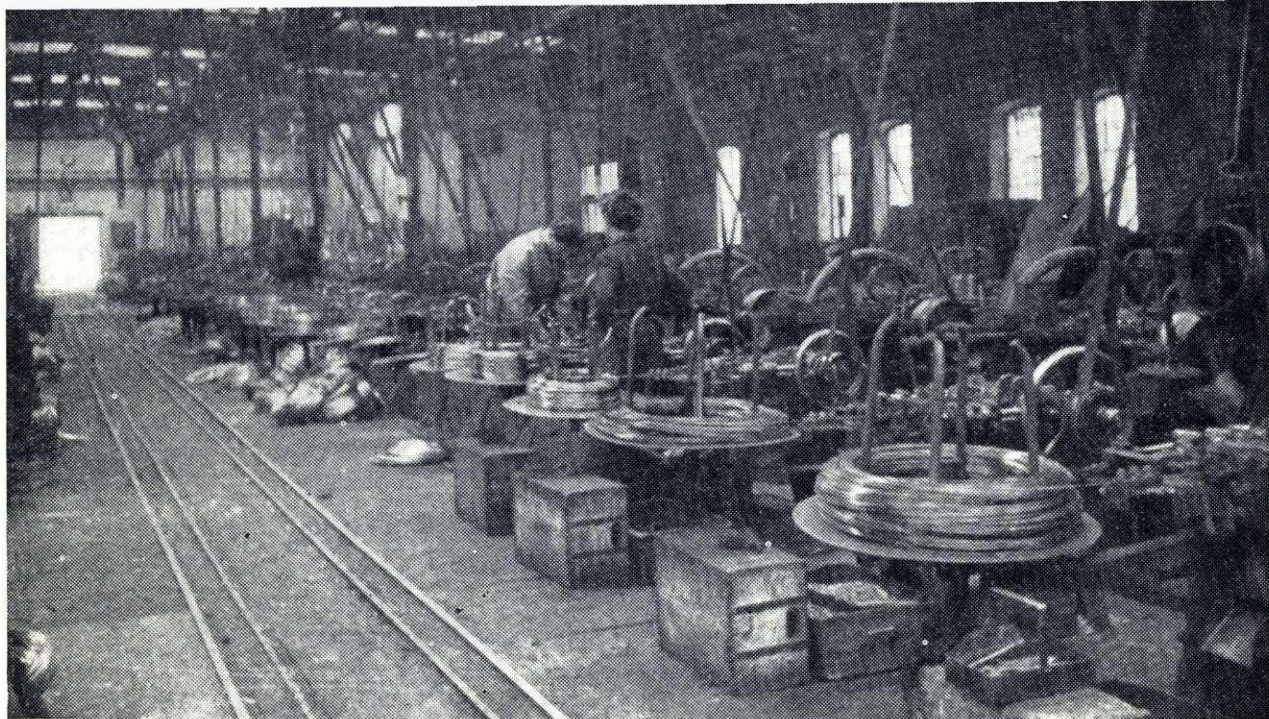
Tako izgleda notranjost naše žebtlarne — Foto Torkar
