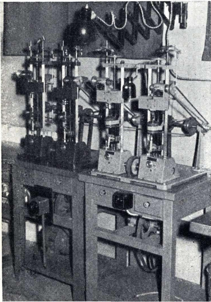
Novi stroji za brušenje diamantov v predelovalnih obratih Foto Torkar
