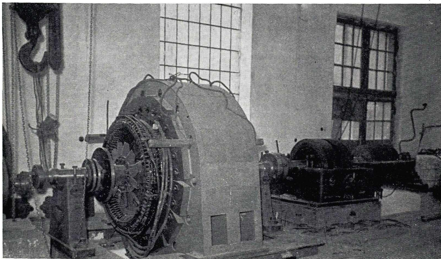
Parna turbina MAN, ki so jo montirali v naši kalorični centrali — Foto France Torkar
