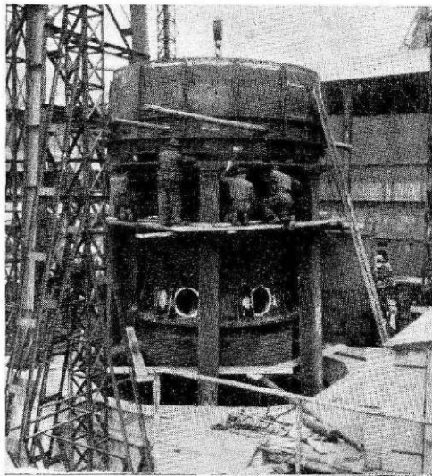
Delo na železnem oklepu novega plavža
