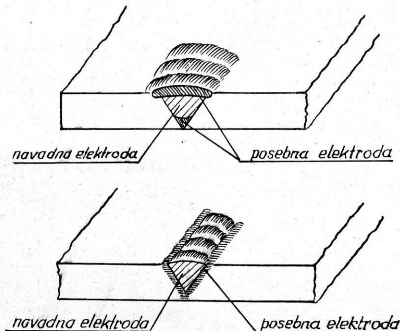
Sl. 18. Mrzlo varjenje litega železa. Štednja pri varjenju z Monelovimi elektrodami
