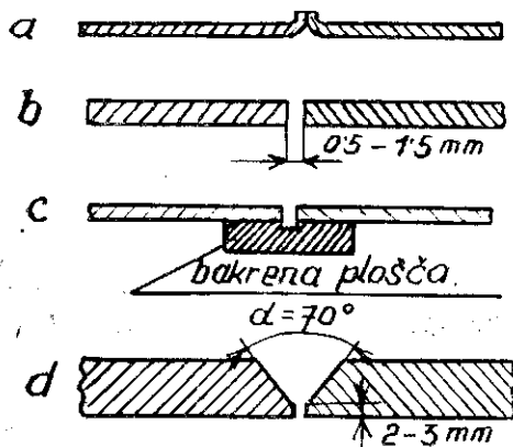
Sl. 4. Priprava topih šivov.
