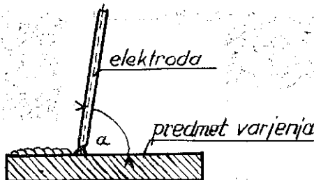
Sl. 2. Drža elektrode.
