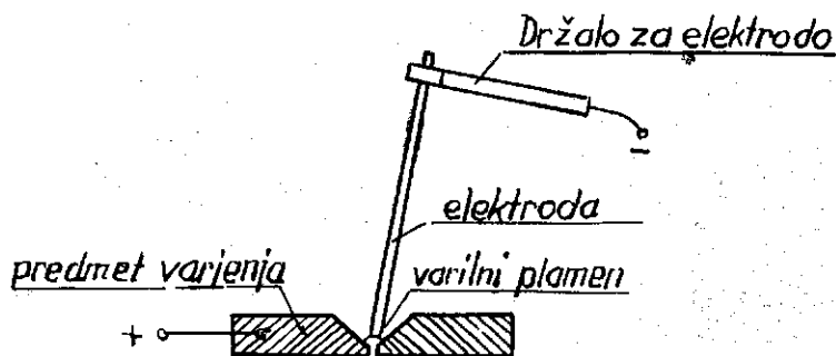
Sl. 1. Shema varjenja po Slavianovu.
