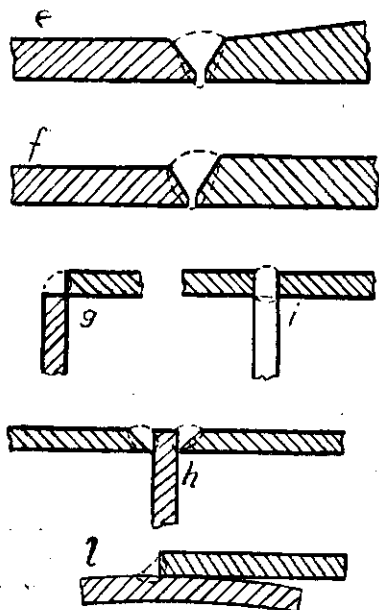
Slika 6: Priprava delov za varjenje
