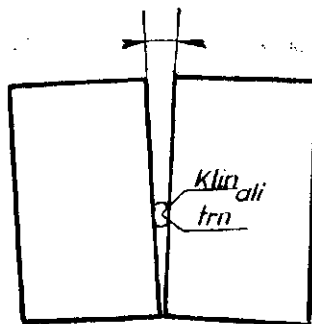
Slika 7. Razširjenje varilne špranje
