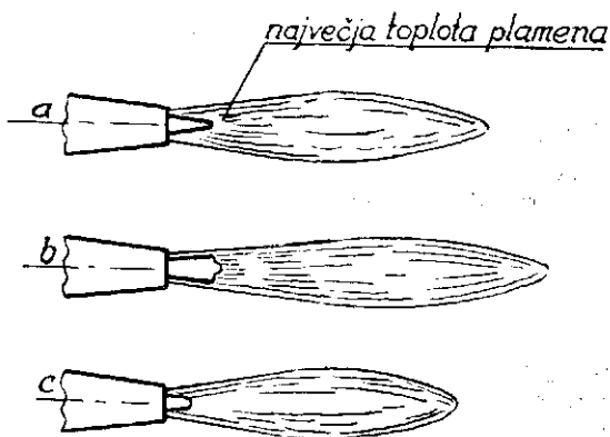
Sl. 3. Uravnavanje varilnega plamena
