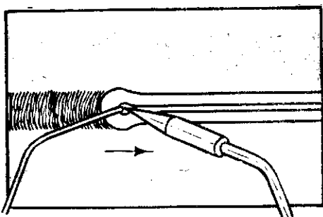
Sl. 5. Shema varjenja na desno
