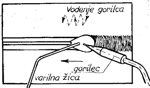
Sl. 4.-Shema varjenja na levo
