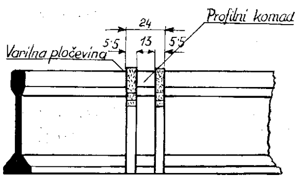
Sl. 2 Varjenje stika tračnic (Elektro-termit)
