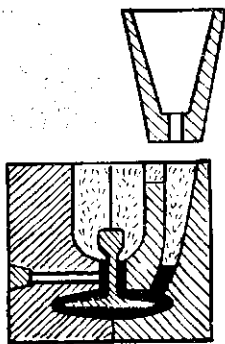
Sl. 1 Shema kombiniranega termitnega varjenja
