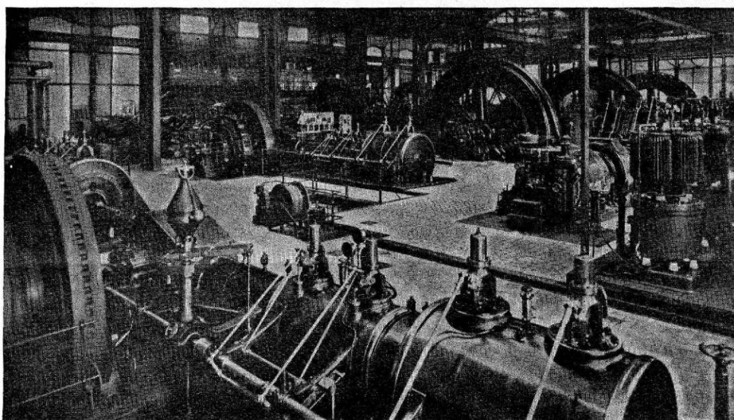
Moderni obrati izkoriščajo plavni plin: Visoke peč. Električna centrala na plin
