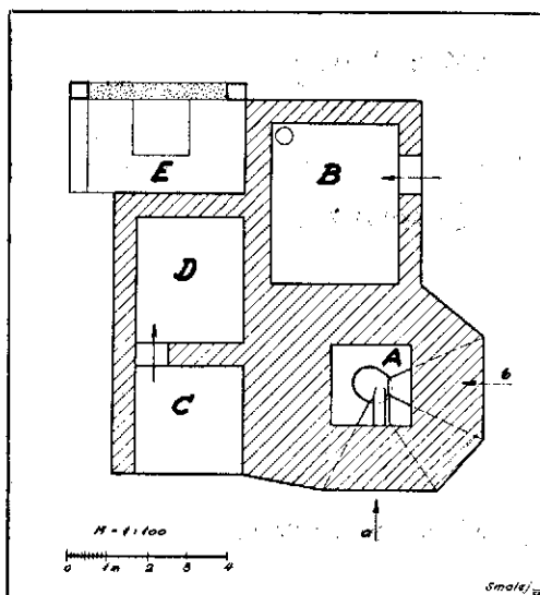
Topilnica sv. Heme pri Nomenju A plavž, B delavnica, C predprostor, D skladišče, E kuhinja
