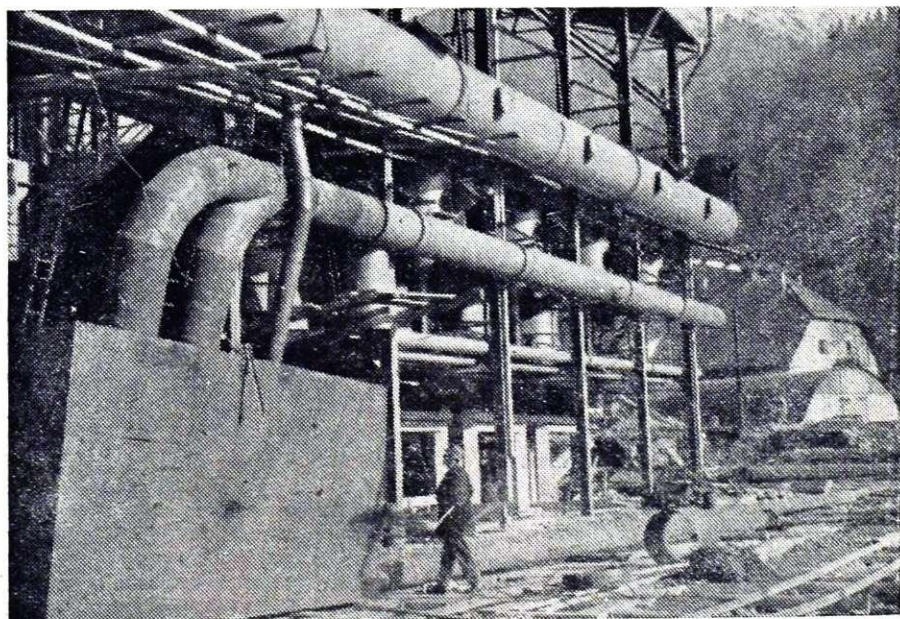
Sodobni novi generatorji za valjarno 2400 na Slovenskem Javorniku
