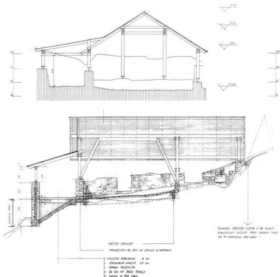
Vzdolžni in prečni prerez končne prezentacije in sistem sanacije zidov
