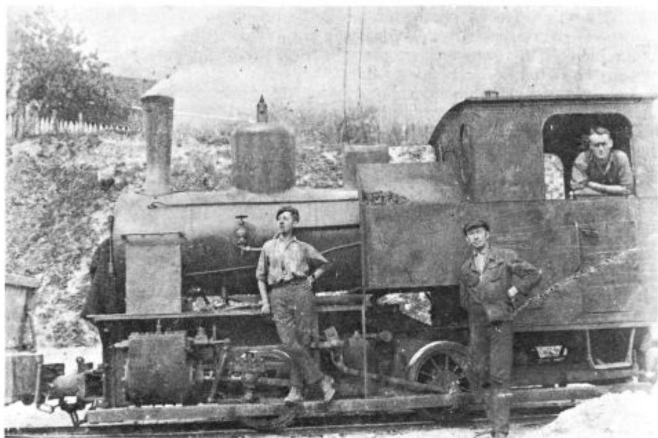
Ozkotirna parna lokomotiva O-II iz leta 1913
