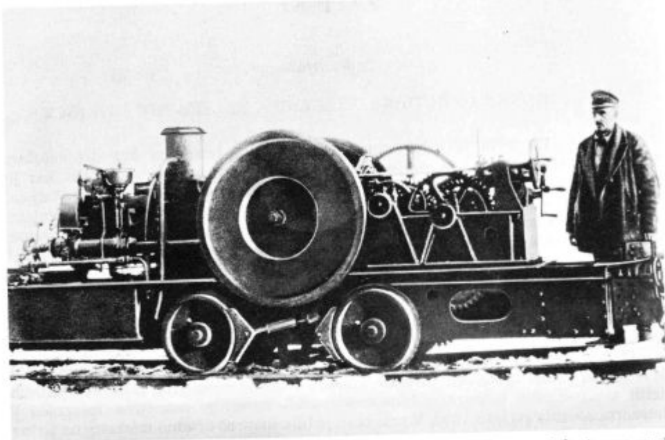
Ozko tirna enocilindrska bencinska lokomotiva (brez ohišja), ki je prevažala tovore med Jesenicami in Javornikom leta 1905. Imenovali so jo tudi »prašič«
