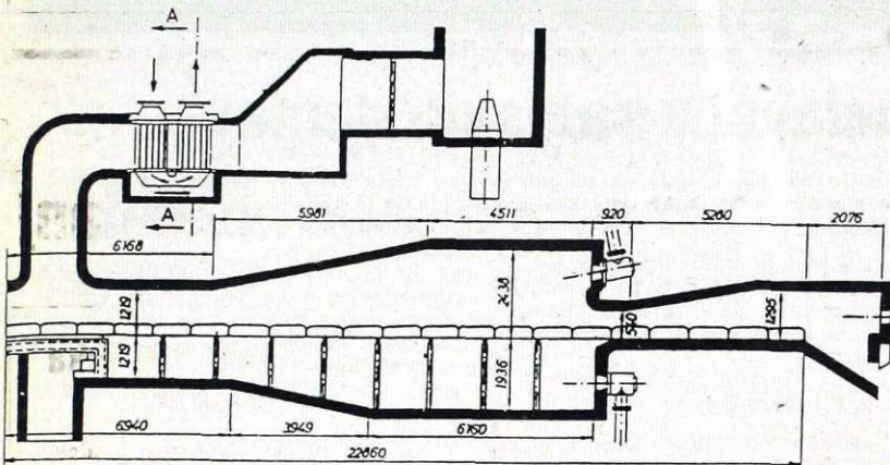
Slika 1: Potisna peč pred rekonstrukcijo
