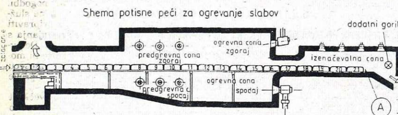
Slika 2: Potisna peč po rekonstrukciji
