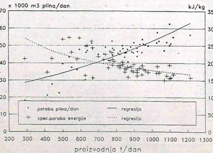
Slika 3: Vpliv storilnosti potisne peči na specifično porabo zemeljskega plina.
