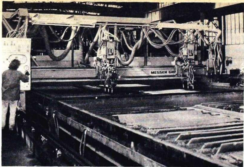
Autogeno rezanje pločevine (foto: Mira Kolenik)
